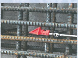
壁配筋の鉄筋のあき 25mmを確認。
