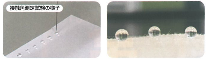
【接触角測定】綿素材を使用し行った場合は超撥水を確認
