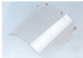
No.3006 取替えレンズ ¥1,600 100980 透明PET樹脂 1.5mm厚×長さ195mm 製品重量:約103g
