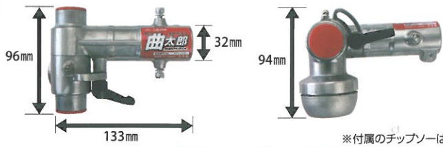
■ 寸法図 (チップソー除く)
