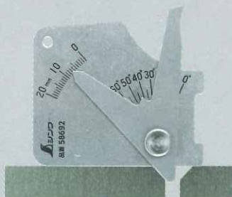
ベベル角度測定
