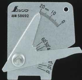
NEW 溶接ゲージ B 軽量・薄型
