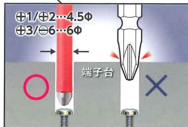
細軸仕様なので、狭い箇所や 穴奥のネジにも対応できます。
