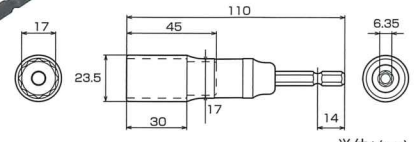
ETS-17SS
