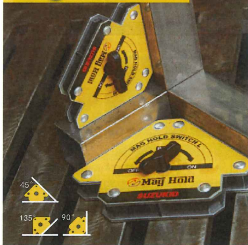
Mag Hold Switch
