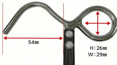
Mサイズ寸法
