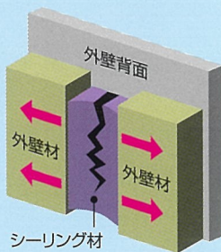
ボンドブレーカーなし
