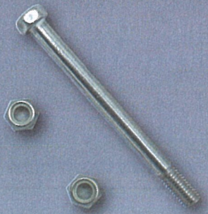
SBN 60 ( 軸ボルト×1 2種ナイロンナット×2 )
