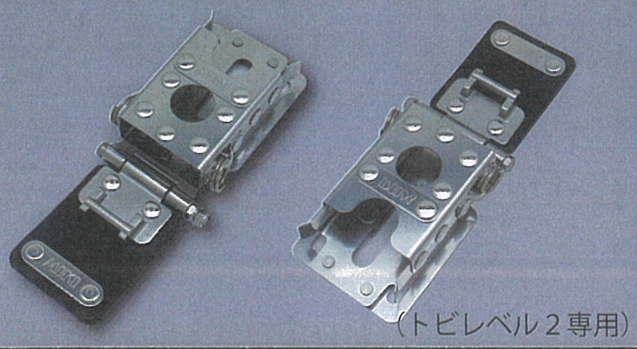
SBN 60 ( 軸ボルト×1 2種ナイロンナット×2 )
